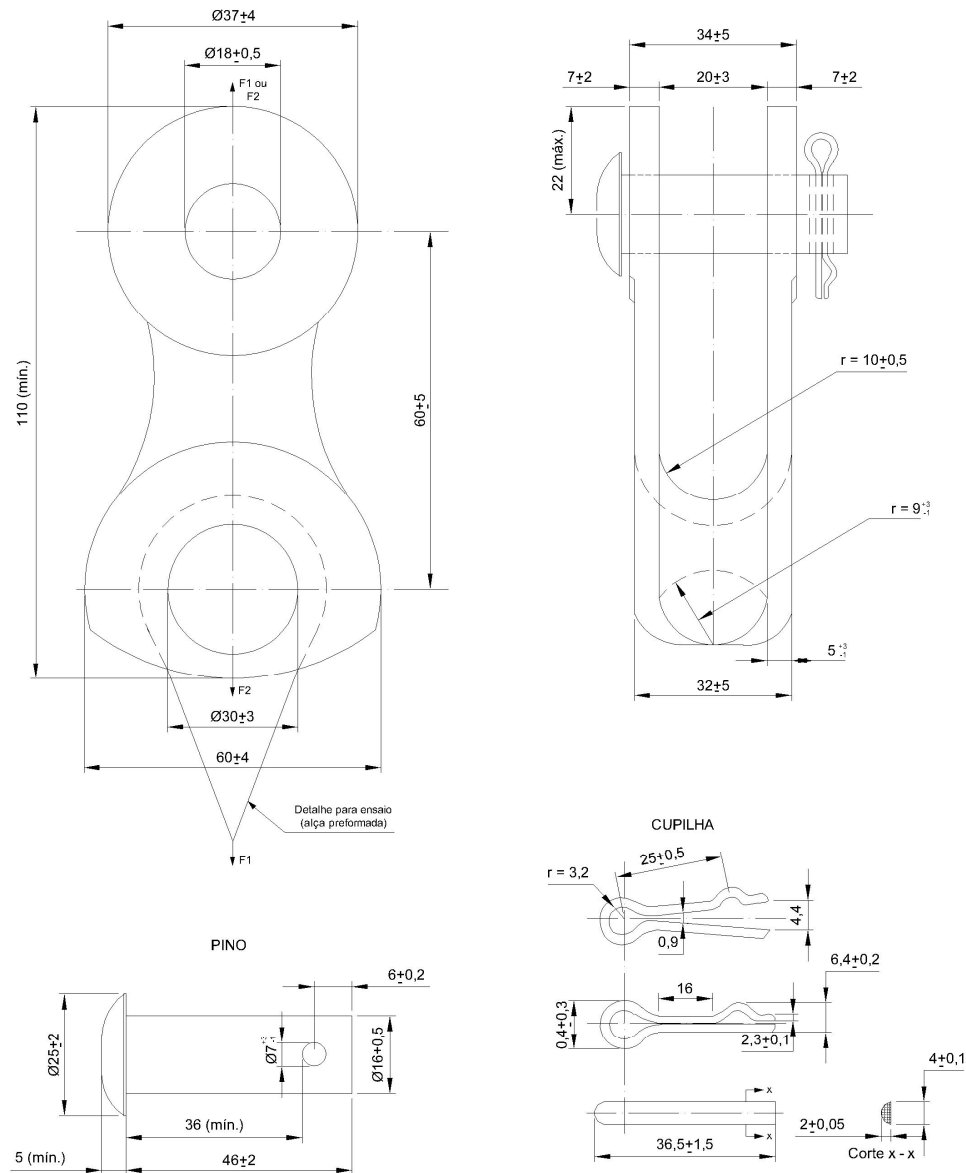
Figura 3 - Desenho dimensional conjunto manilha-sapatilha
