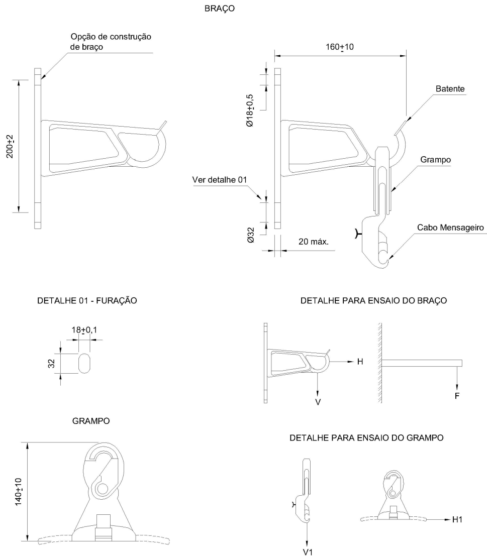
Figura 1 - Desenho dimensional conjunto grampo de suspensão
