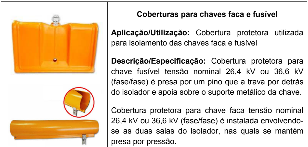
Figura 107 – Coberturas para chaves faca e fusível
