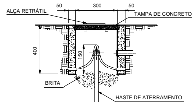
CORTE AA'
